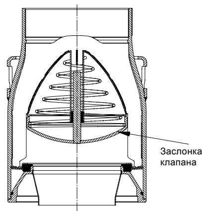
Рис. 5 Обратный клапан
