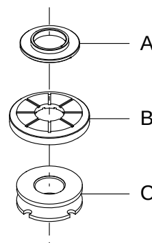
Рис. 7 Стопорное кольцо
