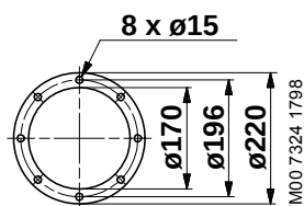
Насос с фланцем Grundfos
