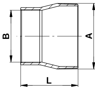
Рис. 31 Габаритный чертеж и изображение соединительной детали резьба-резьба
